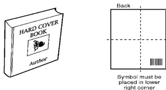
Abbildung 6.4.11-1. Symbolplatzierung auf Büchern
