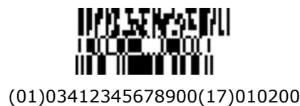
Abbildung 5.11.8-6. GS1 DataBar Stacked Symbol mit einer 2-spaltigen CC-A Komponente
