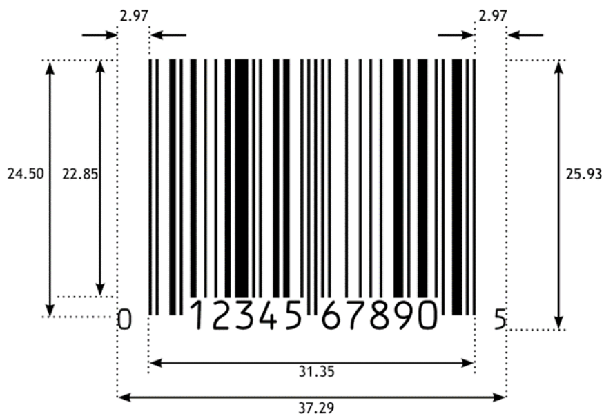
Abbildung 5.2.6.6-2. UPC-A Strichcode
