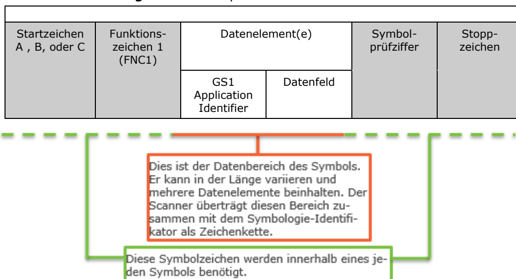
Abbildung 7.8.4-1. Beispiel der GS1-128 Strichcodestruktur
