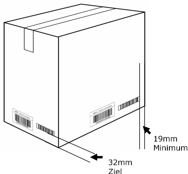
Abbildung 6.7.1.2-1. Symbolplatzierung auf Kartons und Umverpackungen
