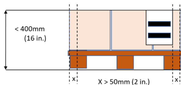
Abbildung 6.7.1.1-2. Symbolplatzierung auf Paletten kleiner als 400 mm (16 inches)
