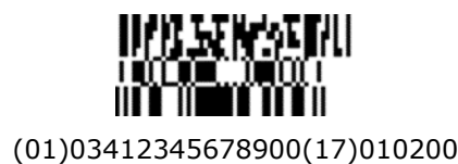
Abbildung 5.9.8-6. GS1 DataBar Stacked Symbol mit einer 2-spaltigen CC-A Komponente
