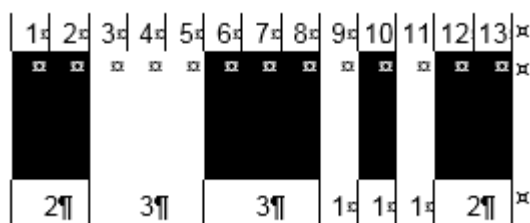
Abbildung 5.4.3.1-3. GS1-128 Stoppzeichen
