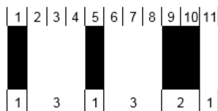
Abbildung 5.4.3.1-2. Symbolzeichenwert 35
