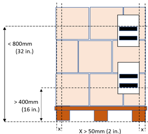
Abbildung 6.7.1.1-1. Symbolplatzierung auf Paletten
