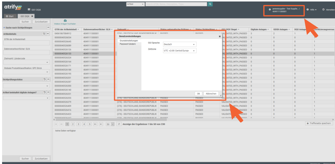
Abbildung 2 – 11: Benutzereinstellungen ändern
