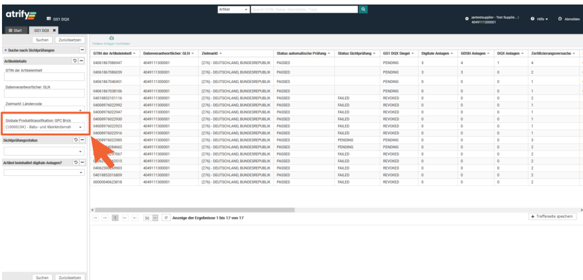
Abbildung 2 – 4: GPC Suche
