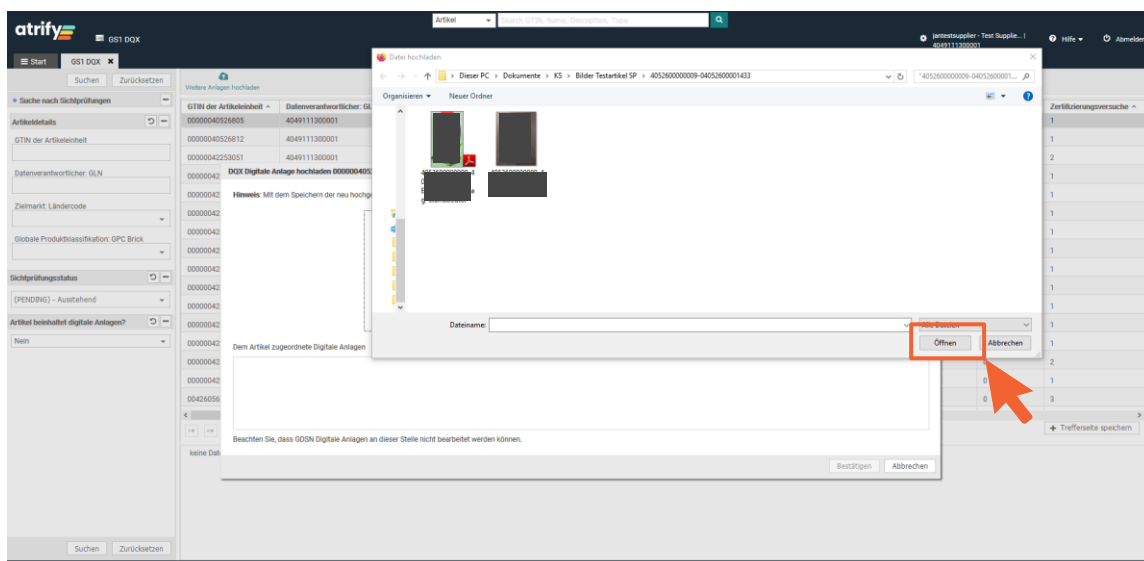
Abbildung 2 – 8: Produktbilder/-artworks hinzufügen
