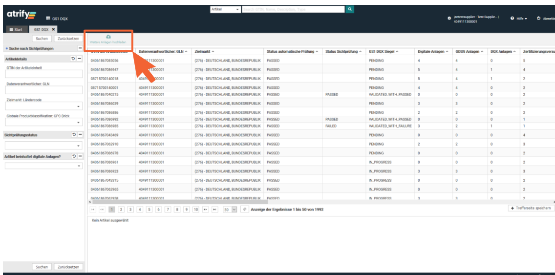
Abbildung 2 – 6: Produktbilder/-artworks hinzufügen
