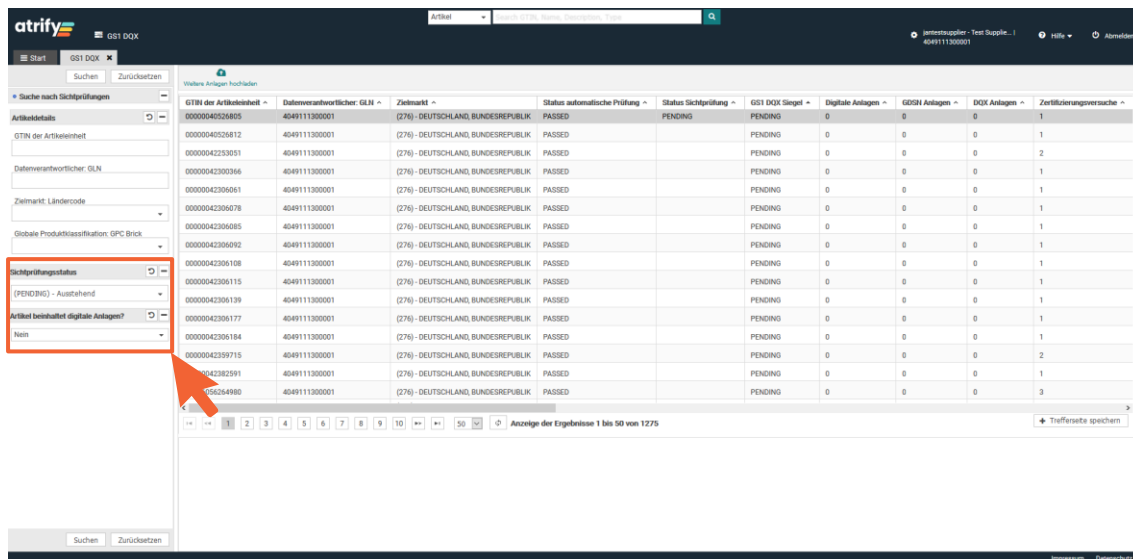
Abbildung 2 – 5: Filter setzen
