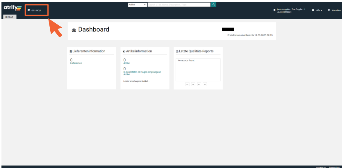
Abbildung 2 – 1: Dashboard
