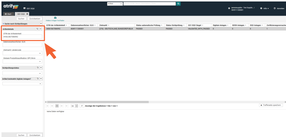
Abbildung 2 – 3: GTIN Suche
