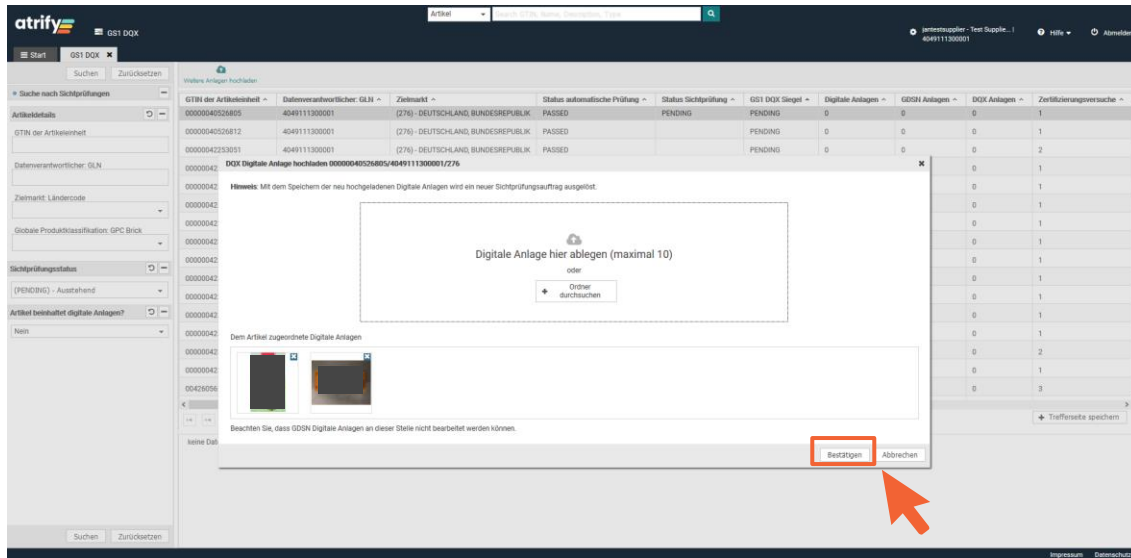
Abbildung 2 – 9: Upload bestätigen
