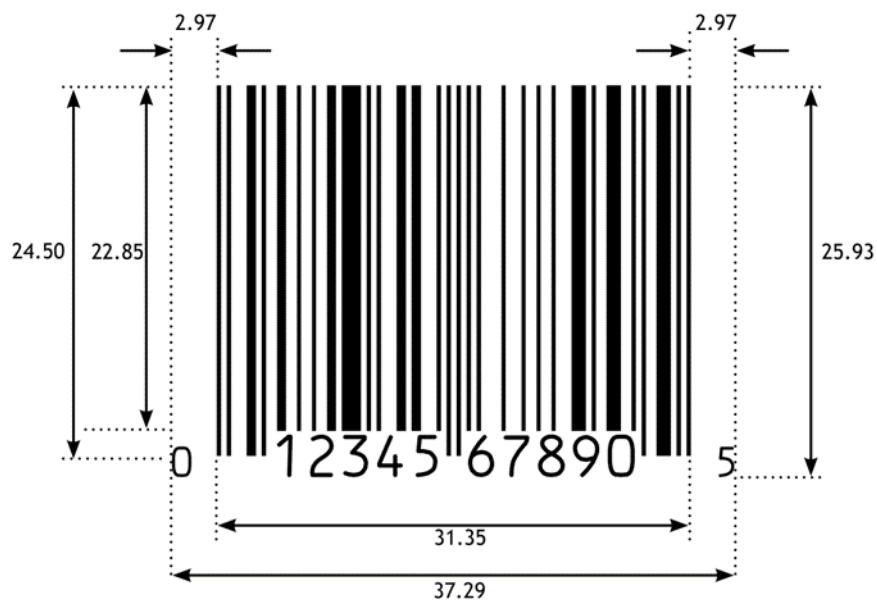
Abbildung 5-24 UPC-A Strichcode
