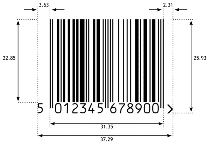
Abbildung 5-23 EAN-13 Strichcode
