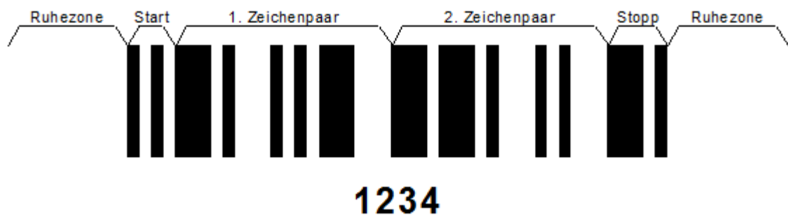
Abbildung 5-31 ITF-14 Symbol einschließlich der Ruhezeiten
