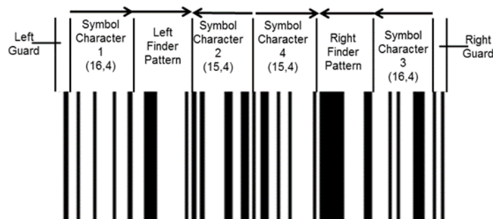
Abbildung 5-39 GS1 DataBar Omnidirectional Struktur
