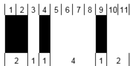
Abbildung 5-35 GS1-128 Startzeichen A
