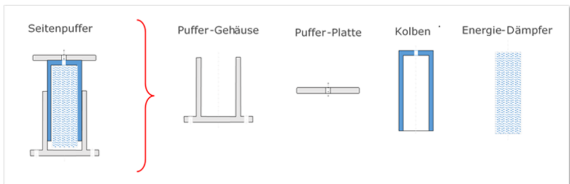
Abbildung 2-4 Beispiel: Puffer (Baugruppe) mit Pufferführung (führendes Bauteil)
