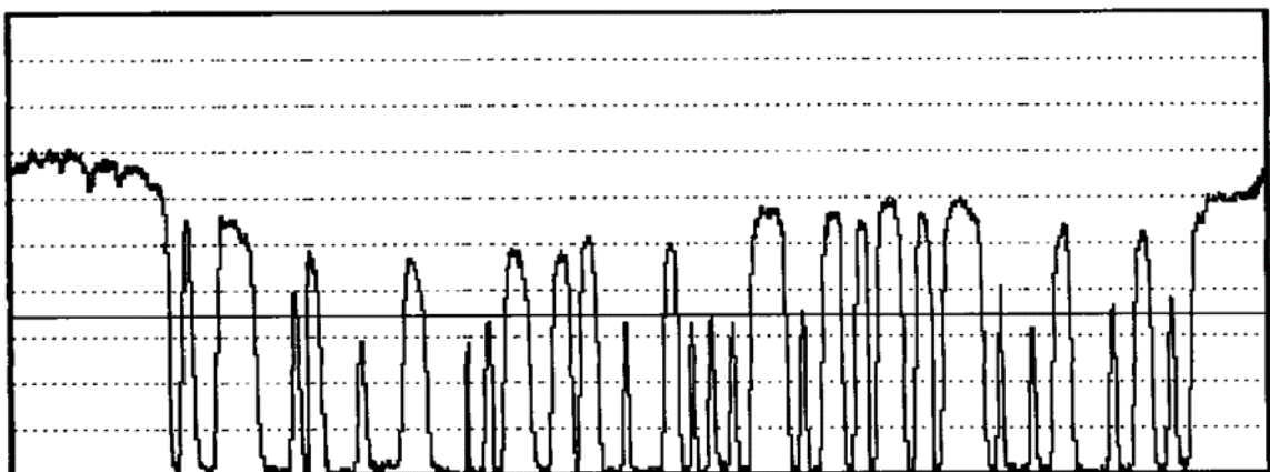
Abbildung 5-72 Scan-Reflexionsprofil mit zu keinen Lücken
