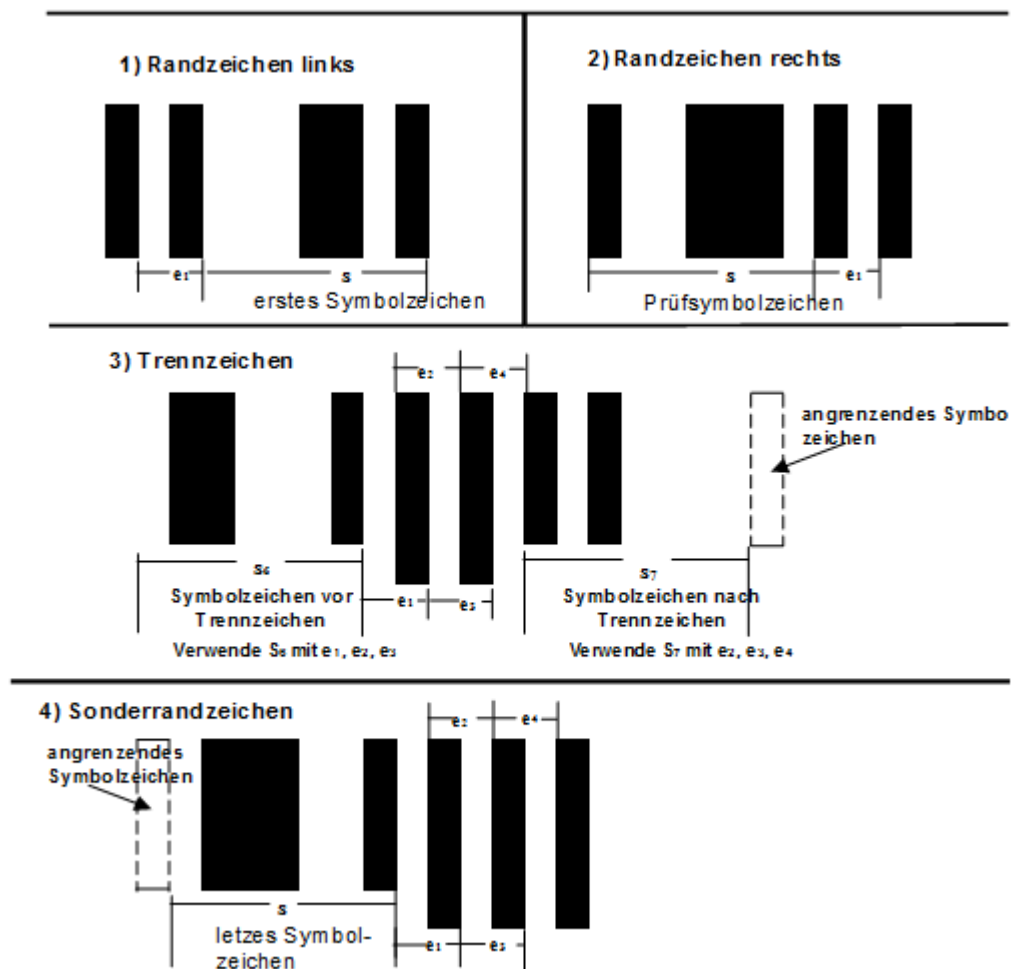
Abbildung 5-22 Messgrößen für EAN/UPC Hilfszeichen
