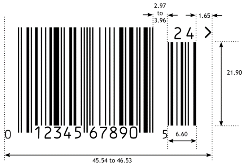
Abbildung 5-27 UPC-A Strichcode mit zweistelligem Zusatzsymbol
