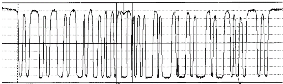
Abbildung 5-74 Scan-Reflexionsprofil eines Symbols mit niedriger Decodierbarkeit
