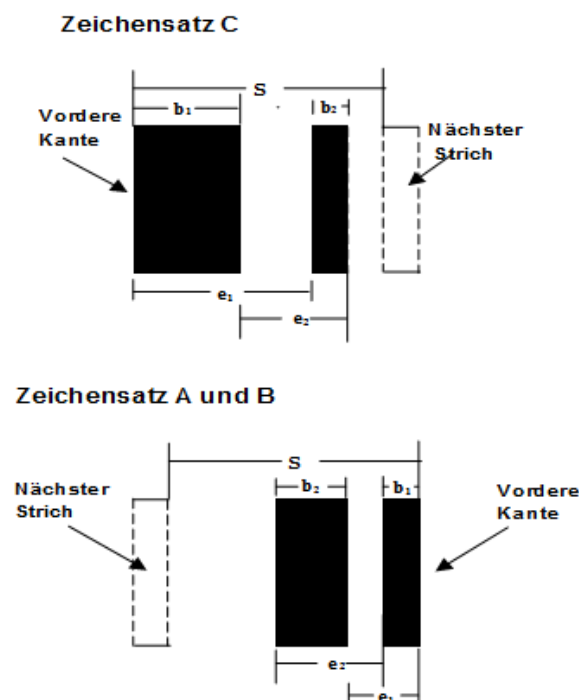
Abbildung 5-21 Messgrößen für ein Symbolzeichen
