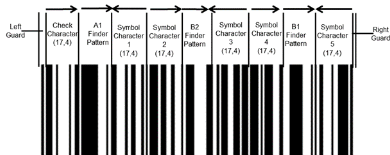
Abbildung 5-46 GS1 DataBar Expanded Struktur
