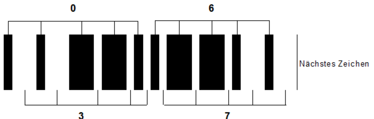
Abbildung 5-29 ITF-14 Zeichenpaar, Verschlüsselung von 03 und 67
