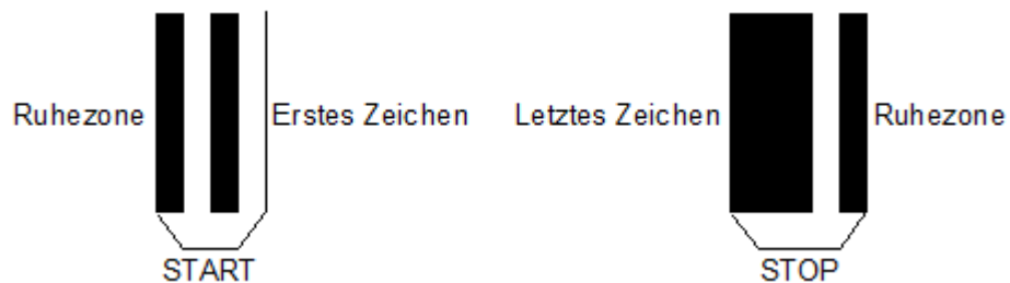
Abbildung 5-30 Start- und Stoppzeichen
