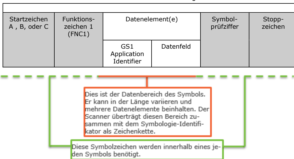
Abbildung 7-8 Beispiel der GS1-128 Strichcodestruktur
